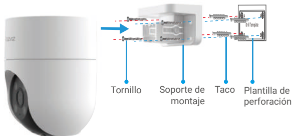
Figura 2. Montaje en pared
