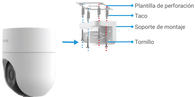
Figura 1. Montaje en techo
